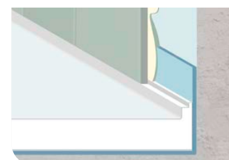
Aufkantung, damit entfällt die Silikonfuge
